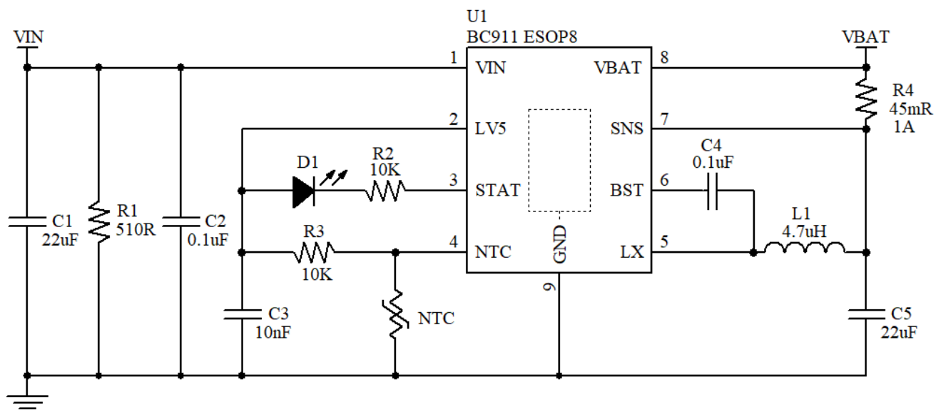
ESOP8 典型应用电路
