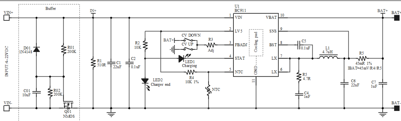
DFN10 详细应用原理图
