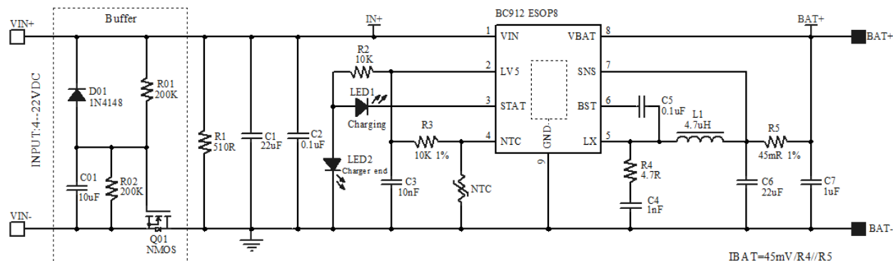
ESOP8 详细应用原理图
