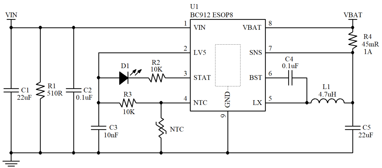
ESOP8 应用电路
