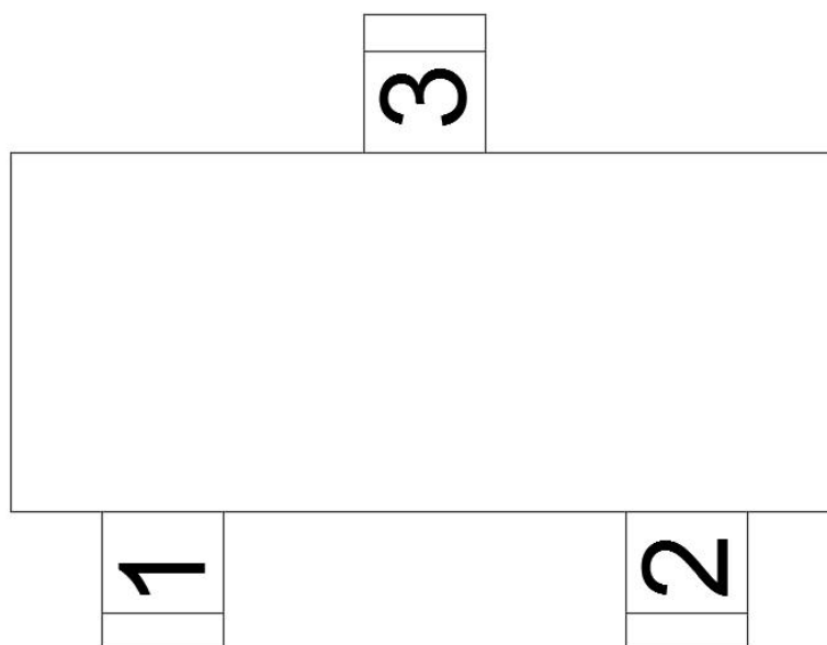
SOT23-3
